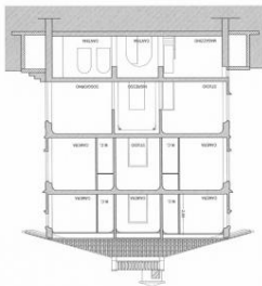
S2 SEZIONE
